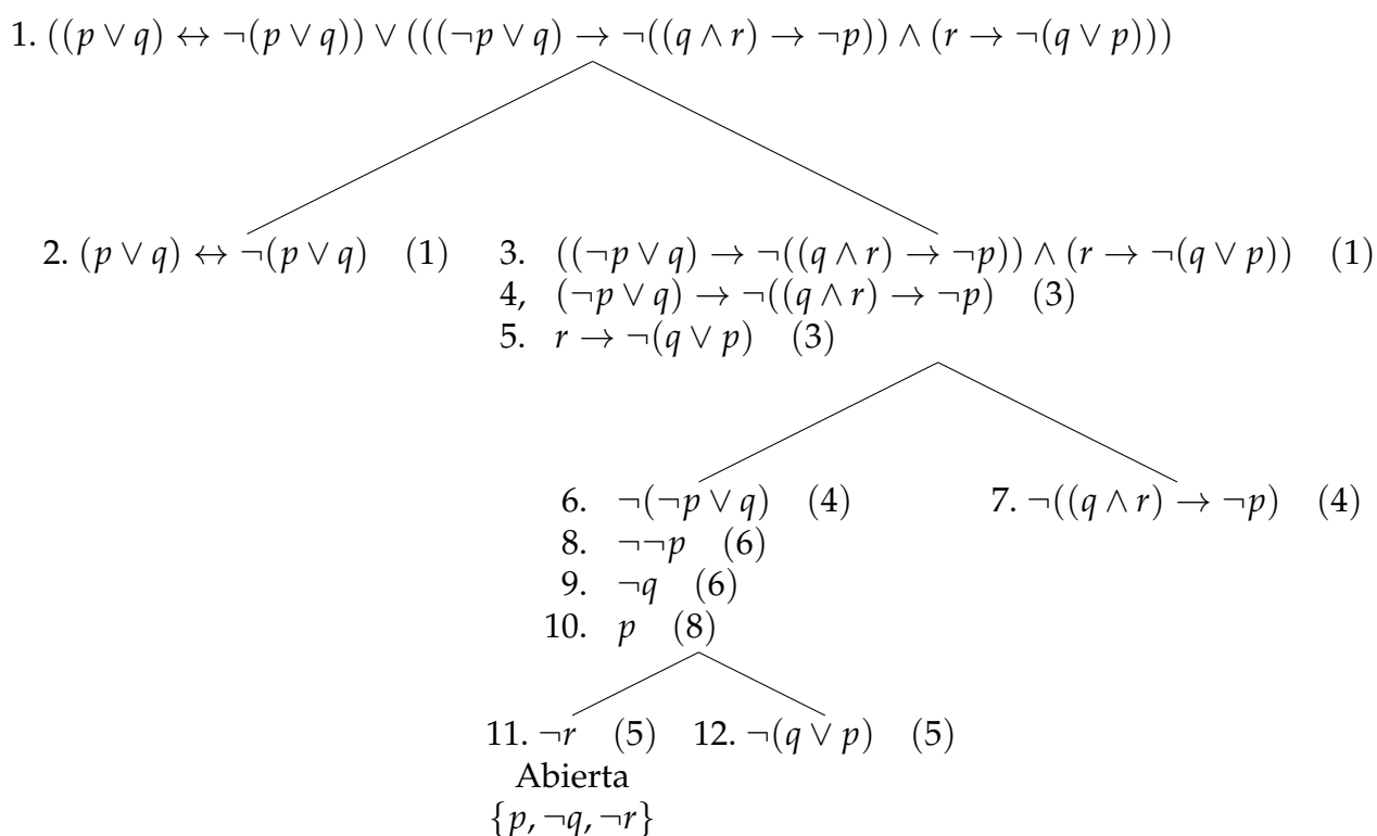
Figura 5: Rama abierta del tablero semántico
